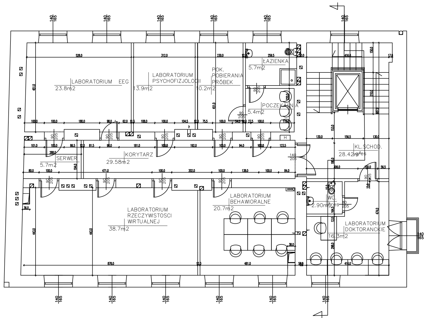
RZUT PIETRA III 1:100
